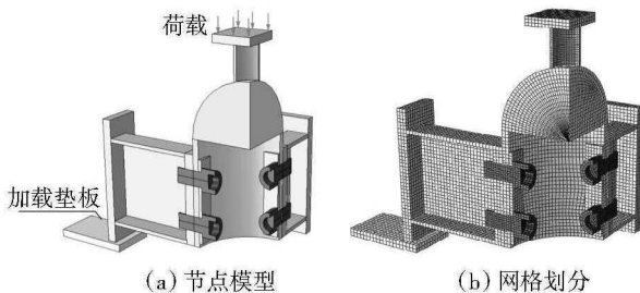
图 3 螺栓球柱节点有限元模型
