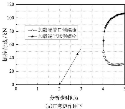
(a)正弯矩作用下
