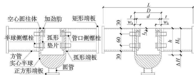
图1 试件详图
