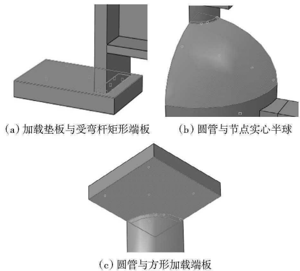
图 4 数值分析模型接触对设置
