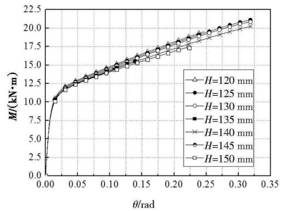
(b)负弯矩作用下 图 16 圆柱筒壁高度的影响
