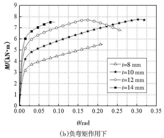
图 17 圆柱筒壁厚度的影响
