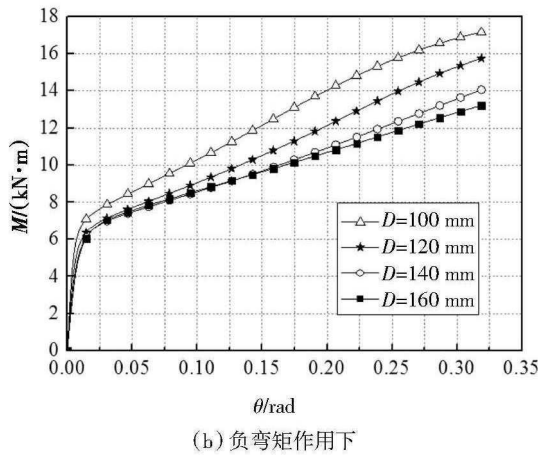
图 15 圆柱筒壁直径的影响
