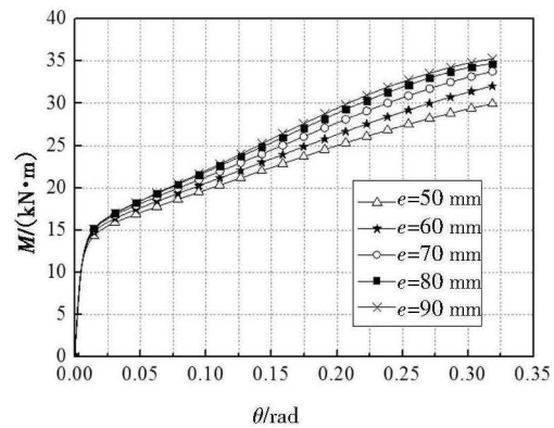
(b)负弯矩作用下
