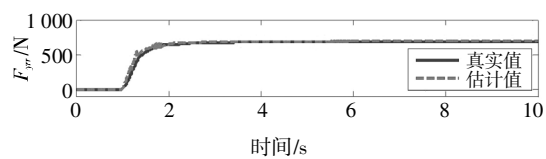
(b)后轴右侧轮胎侧向力
