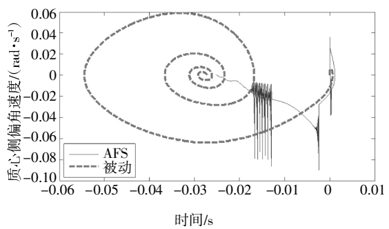
(b)质心侧偏角相平面
